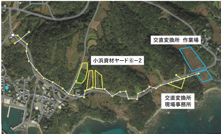
交直変換所配電計画
